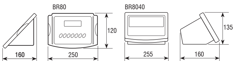
Dimensiones (mm)
