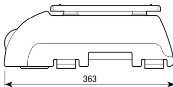
Dimensiones (mm)
