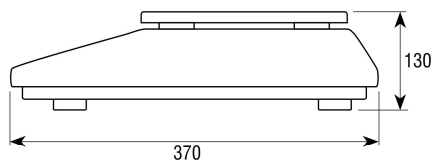
Dimensiones (mm)
